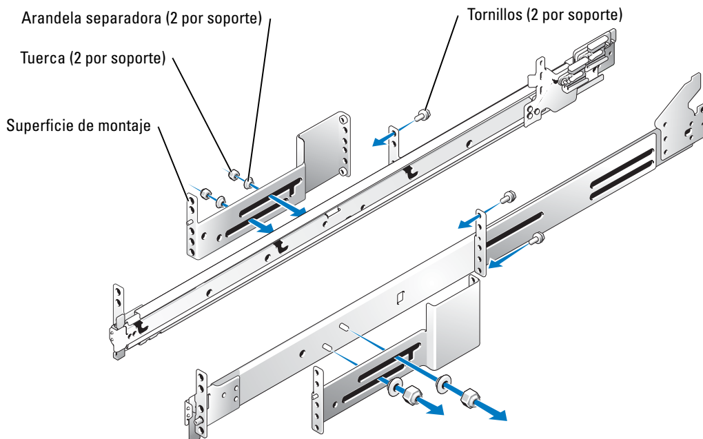
Figura 5-17. Rotación del soporte de montaje frontal para el montaje a ras
