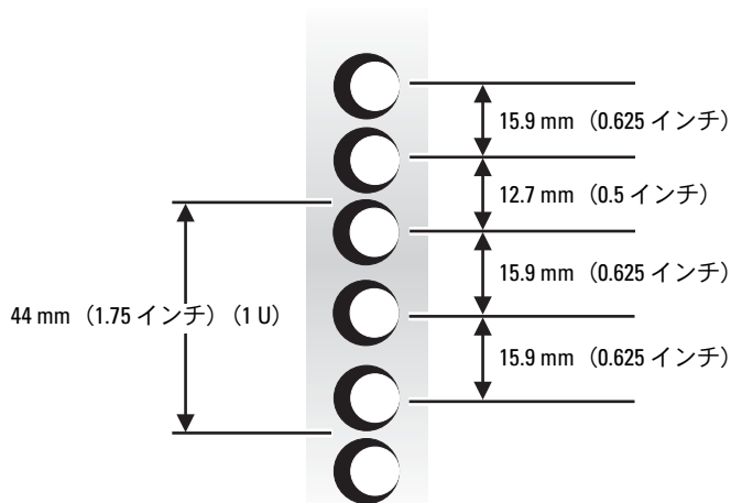
図 4-13 2 柱型オープンフレームリレーラックのユニバーサル間隔の穴
