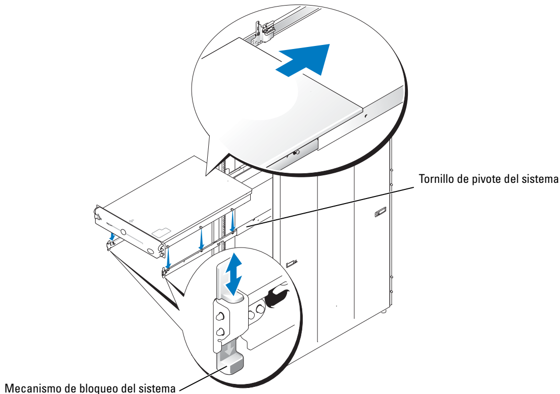
Figura 5-7. Instalación del sistema en el rack (RapidRails o VersaRails)
