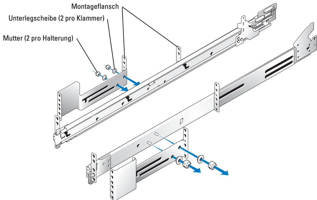
Abbildung 3-15. Klammern für Mittenmontage
