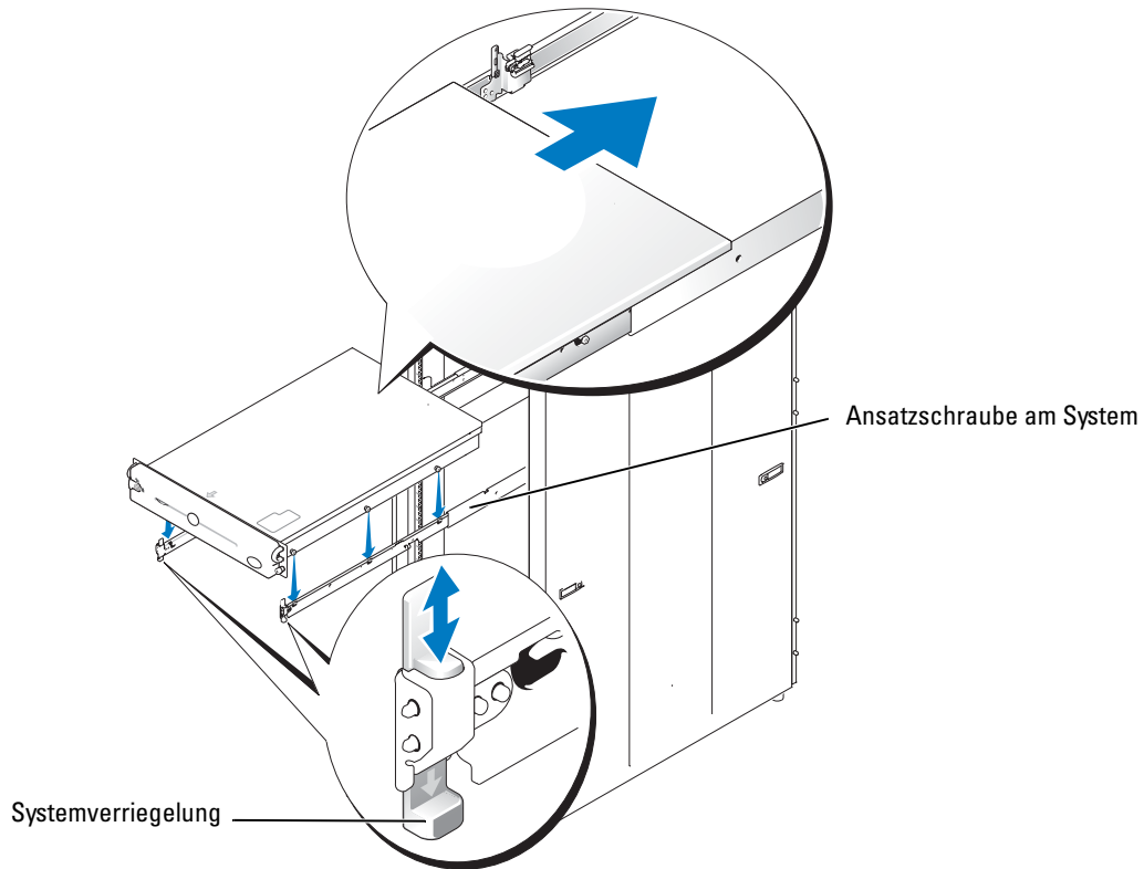
Abbildung 3-7. Installation des Systems im Rack (RapidRails oder VersaRails)
